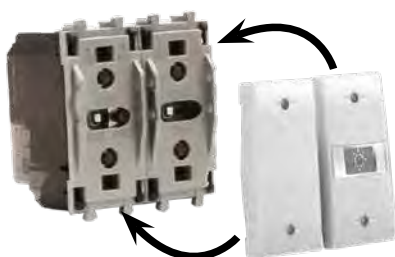
44..ELA01 Tasti 1 funzione 1 function rockers
